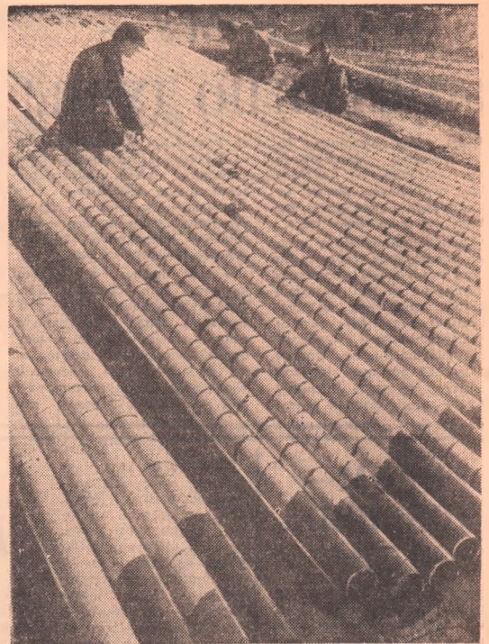
Орское монтажное управление треста «Востокнефтегазпромонтаж». Здесь недавно освоено процесс изготовления усиленной изоляции трубопроводов. Работа эта поручена бригаде слесарей-трубопроводчиков под руководством опытного бригадира Владимира Севастьяновича Штрейса.
