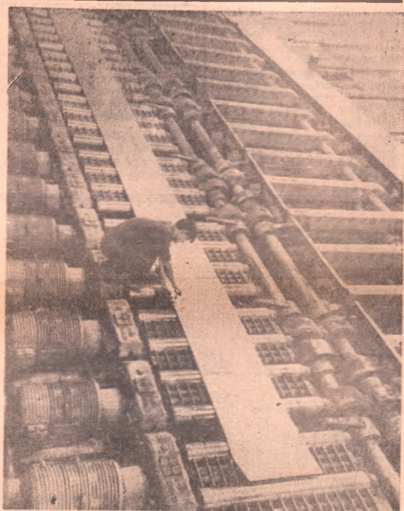
НА СНИМКЕ: новая линия широкого фрезерования в цехе № 2 завода по обработке цветных металлов.
