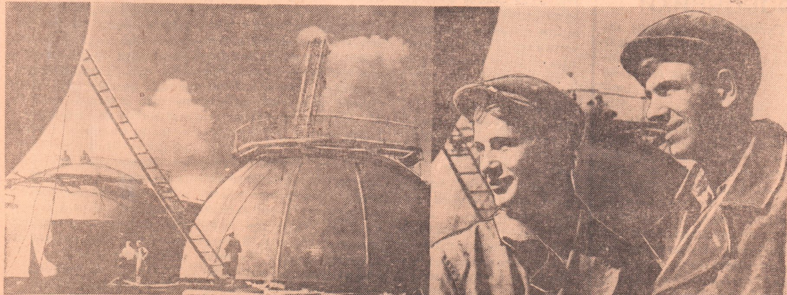
На строительстве новой установки АВТ-ЭЛОУ на заводе имени Чкалова идет сборка корпусов сферических резервуаров. Хорошо трудится на этом участке бригада слесарей-монтажников металлоконструкций из управления «Востокнефтезаводмонтаж», которой руководит Г. Ренна.
