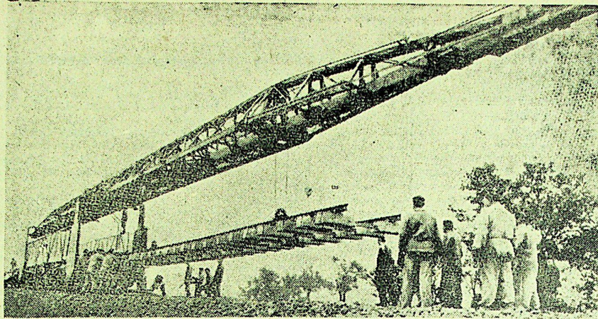
Чехословацкая Социалистическая Республика. На ремонте железнодорожных путей в ЧССР широко используется советская техника. Сроки ремонта при этом значительно сокращаются. На снимке: кран советского производства для укладки рельсов. Фото ЧТК—ТАСС.
