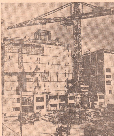
Свердловская область. Строители Белорской атомной электростанции успешно справились с возведением здания реакторного отделения. Сейчас здесь ведутся отделочные работы. Коллектив строится за досрочный сдачу в эксплуатацию первой очереди станции. На снимке: на строительной площадке. Фото П. Лисенкина. Фотохроника ТАСС.
