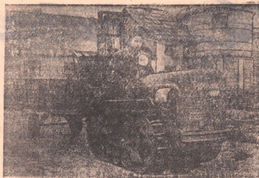
Московская область. В совхозе «Горки-11» проводится производственные испытания малогабаритного трактора «ДТ-16», изготовленного Харьковским тракторным заводом. Новый трактор предназначен для механизации трудоемких работ на животноводческих фермах. Он обладает высокой проходимостью, хорошей маневренностью, может работать с рядом механизмов и приспособлений и производит очистку скотных дворов, подвозку кормов животным и т. д. На снимке: трактор «ДТ-16» с саморазгружающейся тележкой для перевозки удобрений и других грузов. Фото Г. Никитина. Фотохроника ТАСС.
