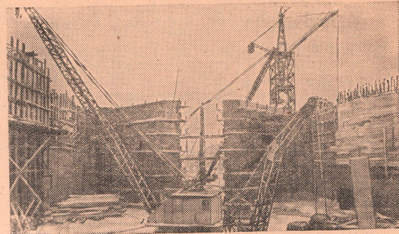
На всех участках строительства Горьковской ГЭС ширится соревнование за досрочную сдачу гидротехнических сооружений в эксплуатацию. На площадке наступают предпусковой период. Полным ходом идет подготовка к перекрытию русла Волги.
